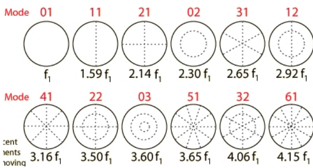
Figure 70: Ütődob-módusok és sajátfrekvenciáik
