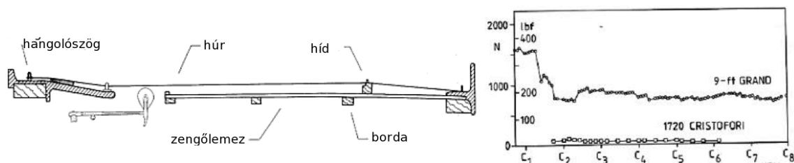
Figure 53: Balra: zongorahúr környezetének keresztmetszete; jobbra: húrok feszítése
