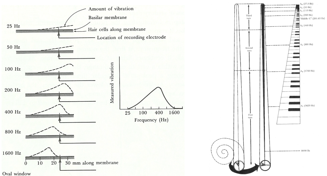
Figure 17: Baloldal: Békésy-féle hullámforma; jobboldal: hangmagasságok érzékelése az alapmembrán mentén.
