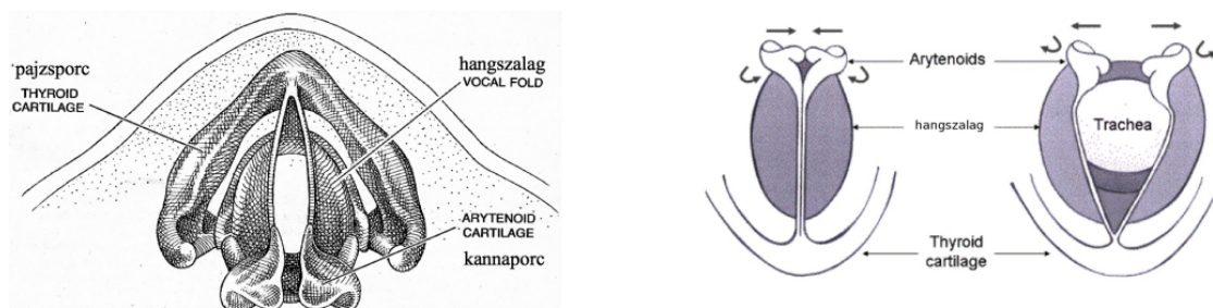
Figure 49: Balra: hangszalag; jobbra: hangszalag zárása-nyitása
