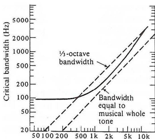
Figure 24: Baloldal: kritikus sávok; jobboldal: hangerőség-sávszélesség összefüggés
