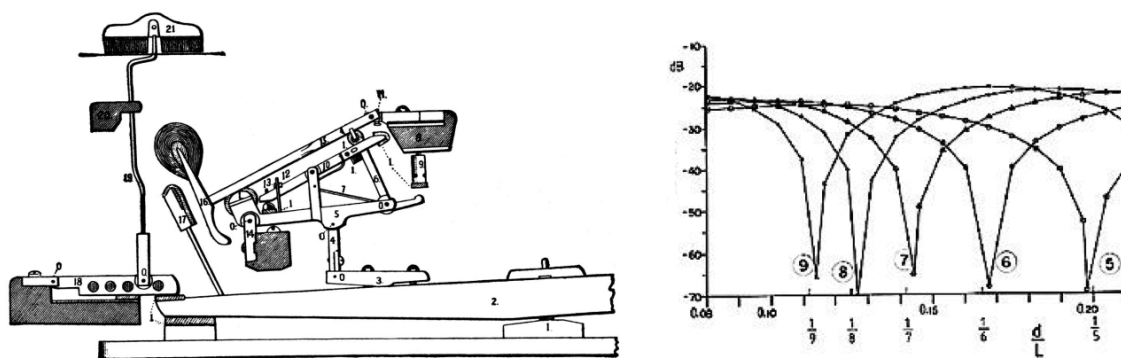
Figure 54: Balra: kalapácsmechanika; jobbra: húr megütési helye
