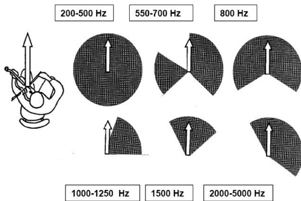
Figure 66: A hegedű iránykarakterisztikája
