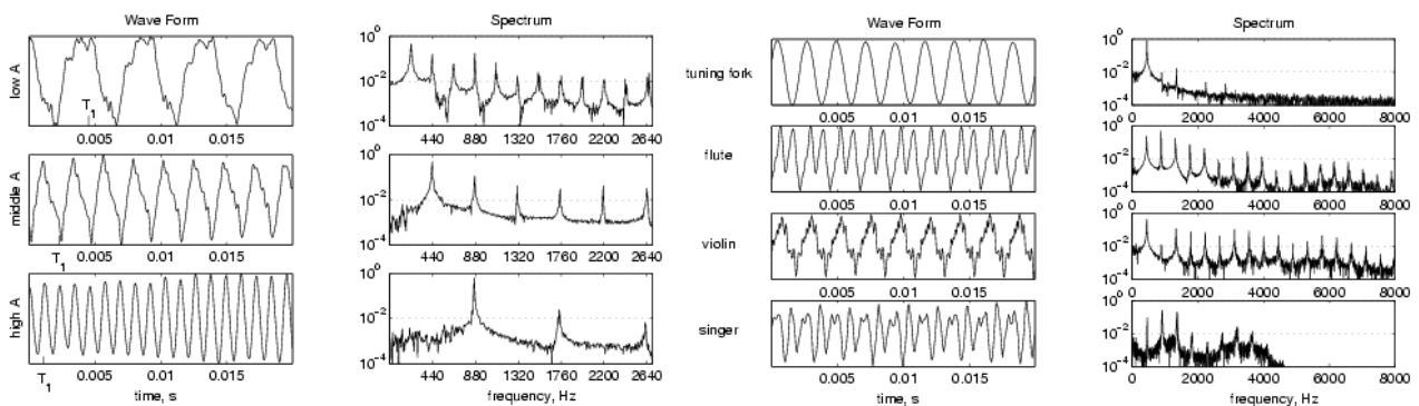
Figure 3: Hullámformák és spektrumaik összehasonlítása. Első oszlop: zongora kis a, a', és a'' hang hullámformája; második oszlop, ugyanezek spektrumaik; harmadik oszlop: kis a hang hullámformája hangvillán, fuvolán, hegedűn, énekhangon; negyedik oszlop: ugyanezek spektrumaik.
