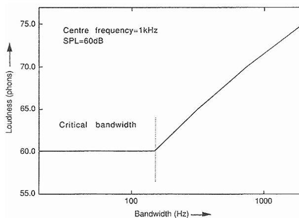
Figure 24: Baloldal: kritikus sávok; jobboldal: hangerőség-sávszélesség összefüggés
