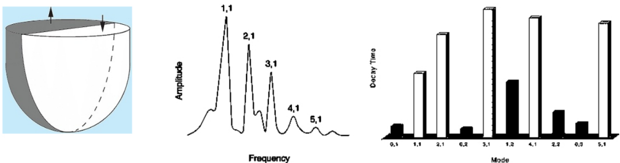
Figure 71: Baloldal: az (1,1) módus; közepén: radiális módusok frekvenciái; jobboldal: radiális (fehér) és cirkuláris (fekete) módusok lecsengési idői.
